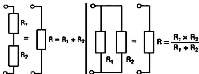
Последовательное и параллельное соединение резисторов
