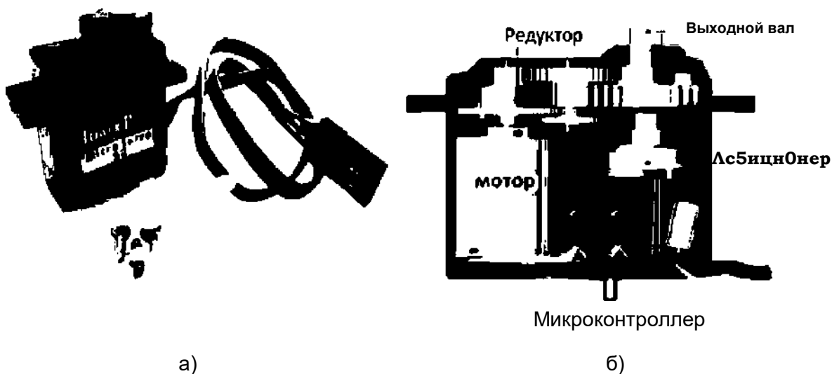
Рис. 2. Сервопривод (а) и его устройство (б)
