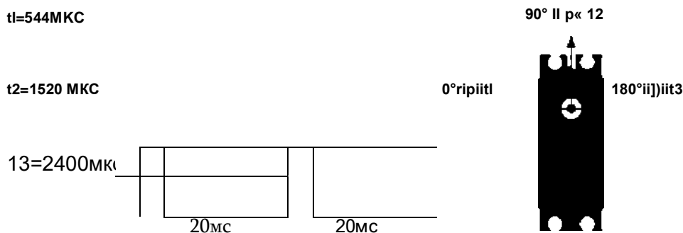
Рис. 3. Схема работы встроенного потенциометра
