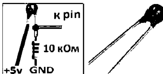
Рис. 3. Схема подключения к микроконтроллерной плате терморезистора
