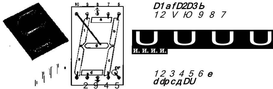
Рис. 13. Семисегментный индикатор и его распиновка
