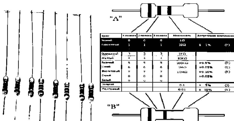
Рис. 6. Резисторы
